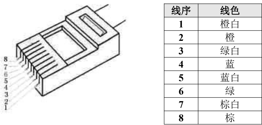
图 1 568B 网线接线线序
